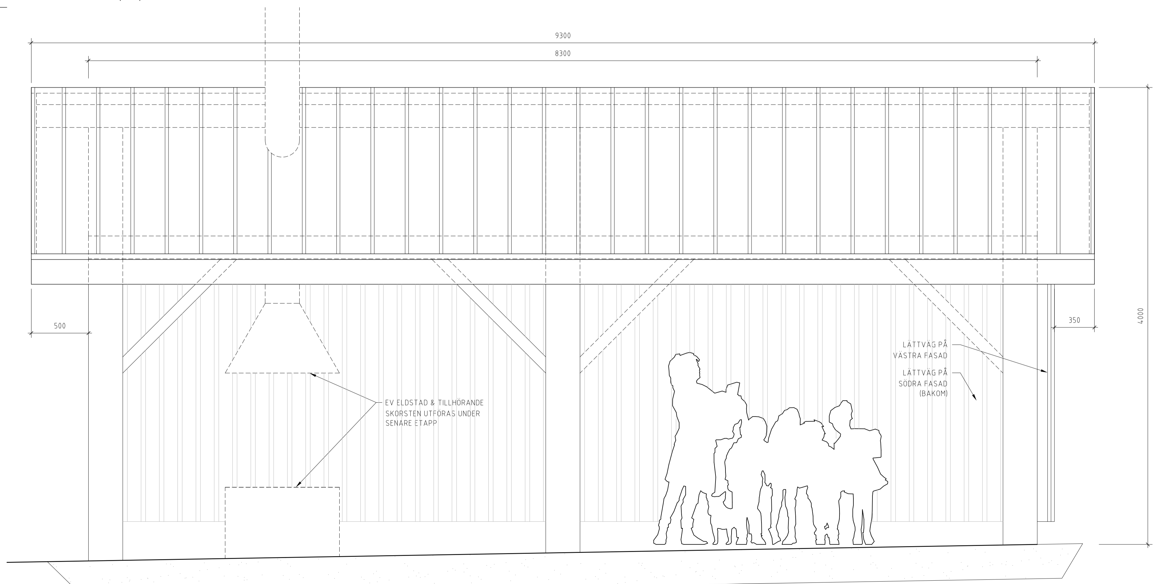
PRINCIP ELEVATION -NORR SKALA 1:20 (A1)
