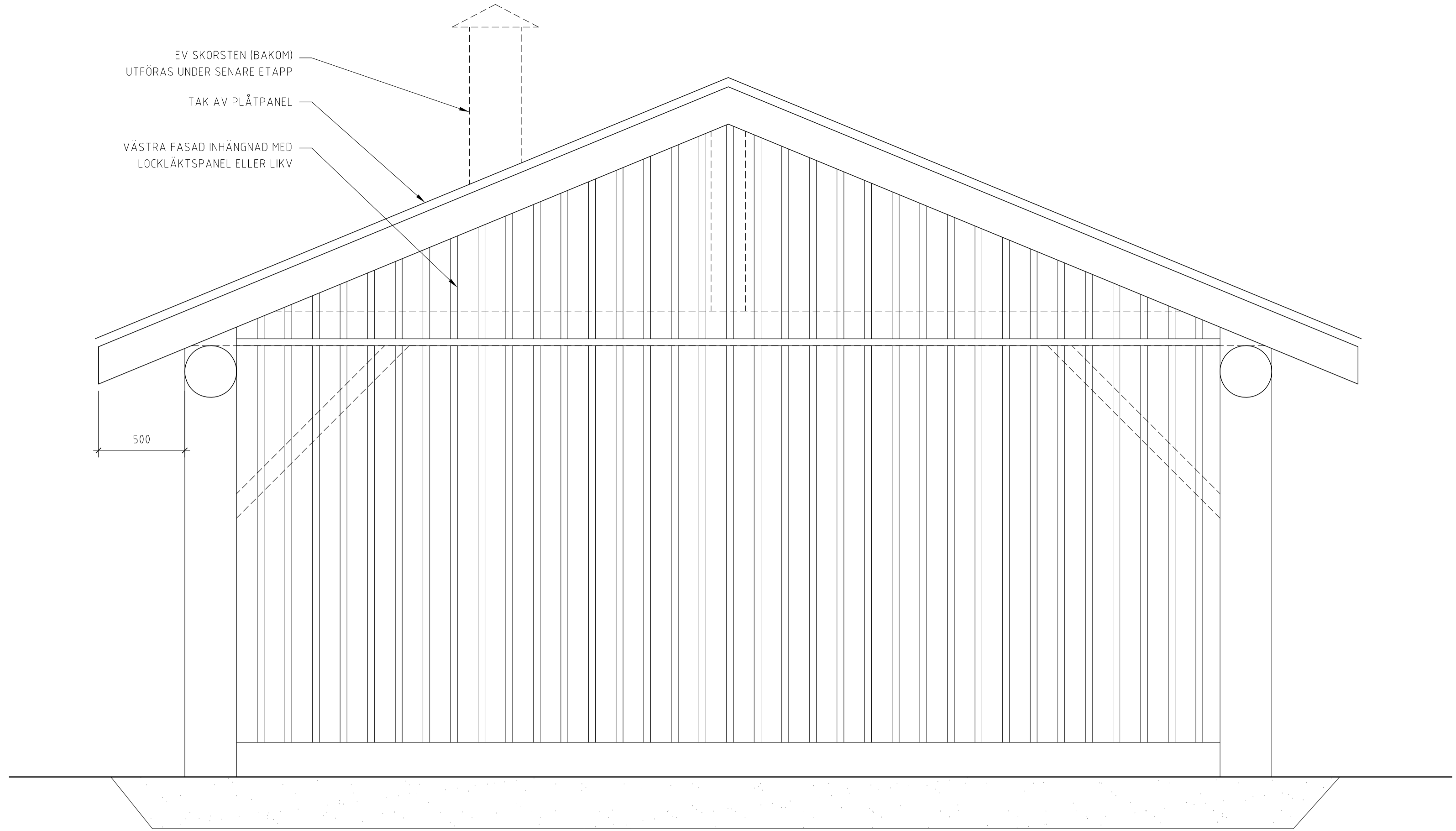
PRINCIP ELEVATION -VÄST SKALA 1:20 (A1)
