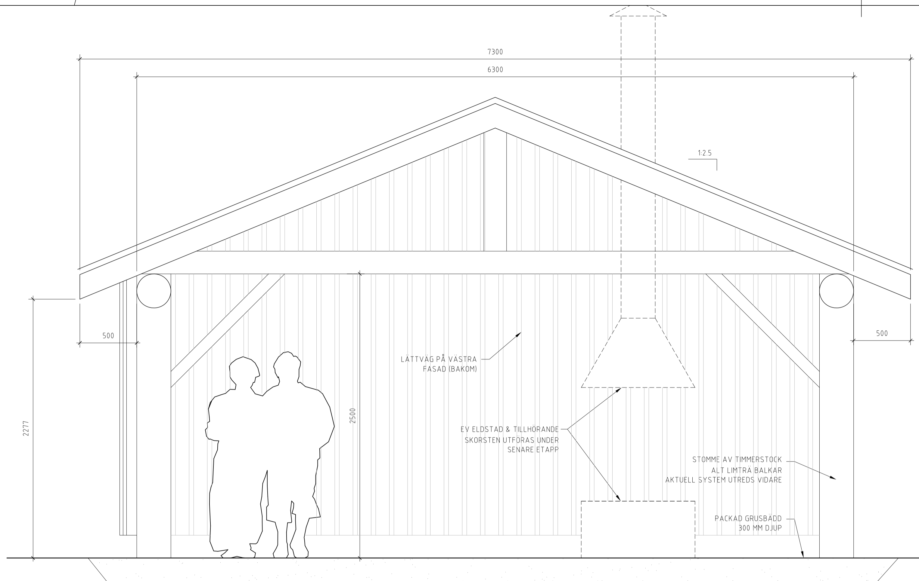
PRINCIP ELEVATION -ÖST SKALA 1:20 (A1)
